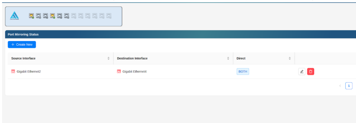
Hình 17: Giao diện hiển thị thông tin cấu hình Port Mirroring
