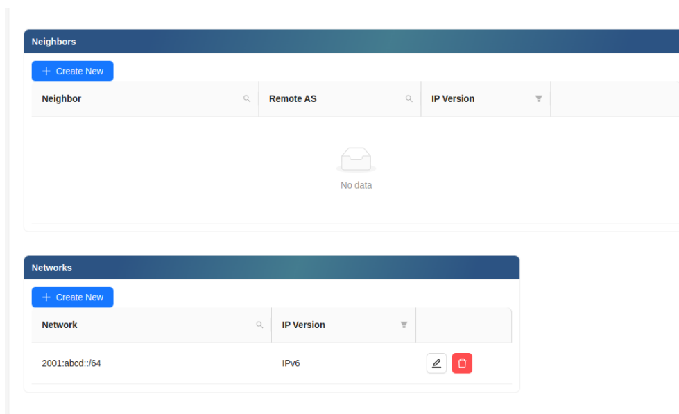
Hình 46: Giao diện thông tin vùng định tuyến trên NGFW theo định tuyến BGP
